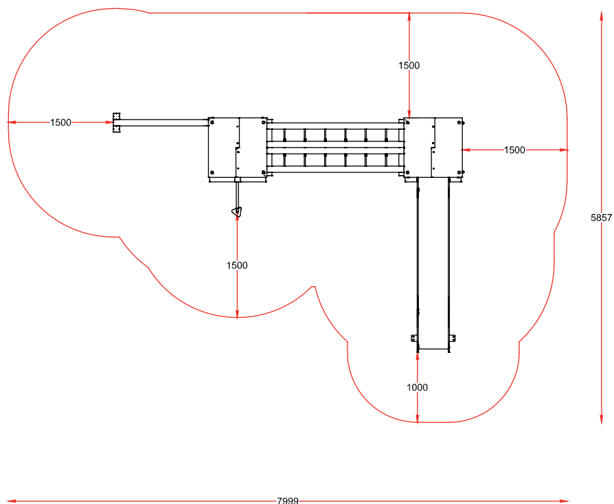
PLANTA
