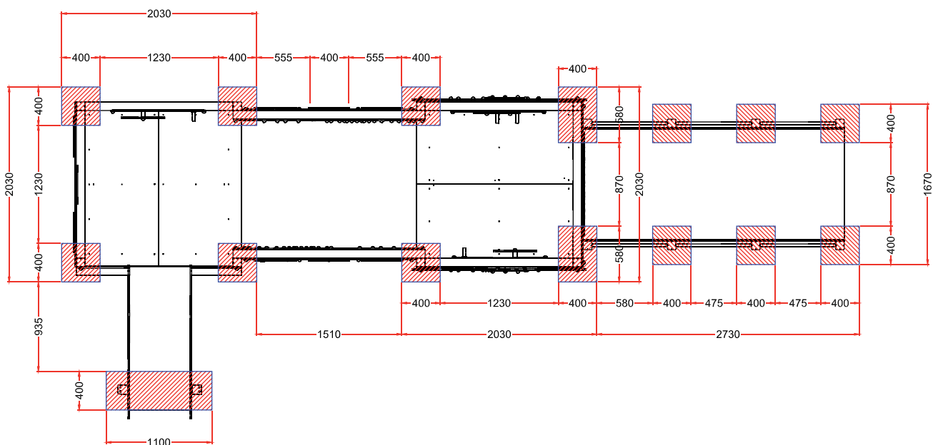
PLANTA CIMENTACION
