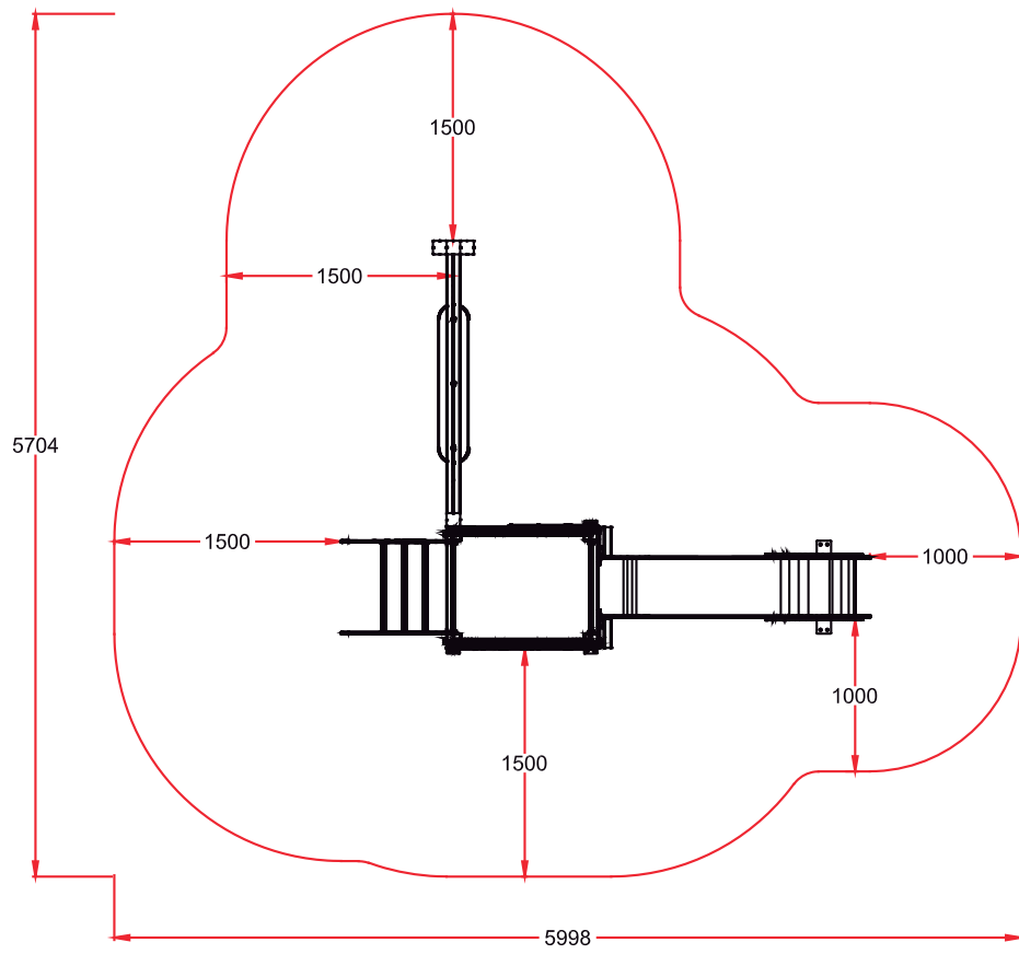
PLANTA
