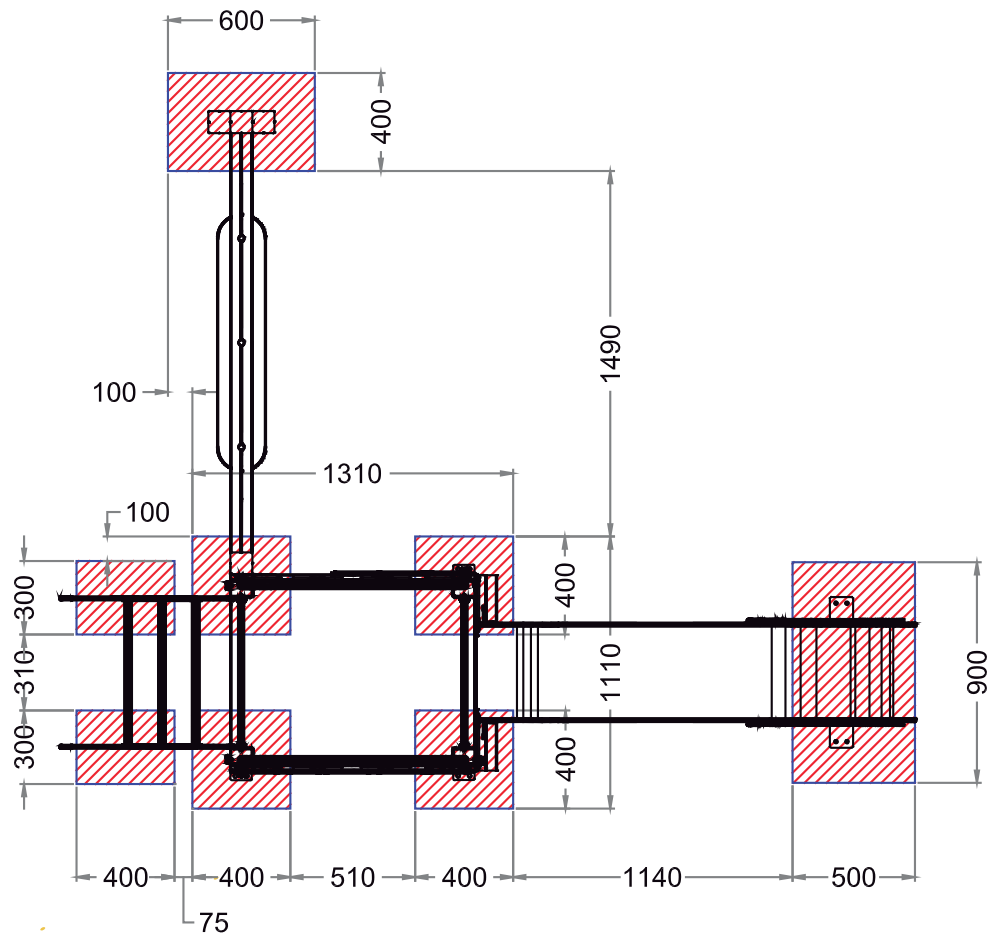
PLANTA CIMENTACION
