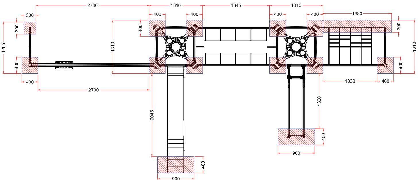
PLANTA CIMENTACION
