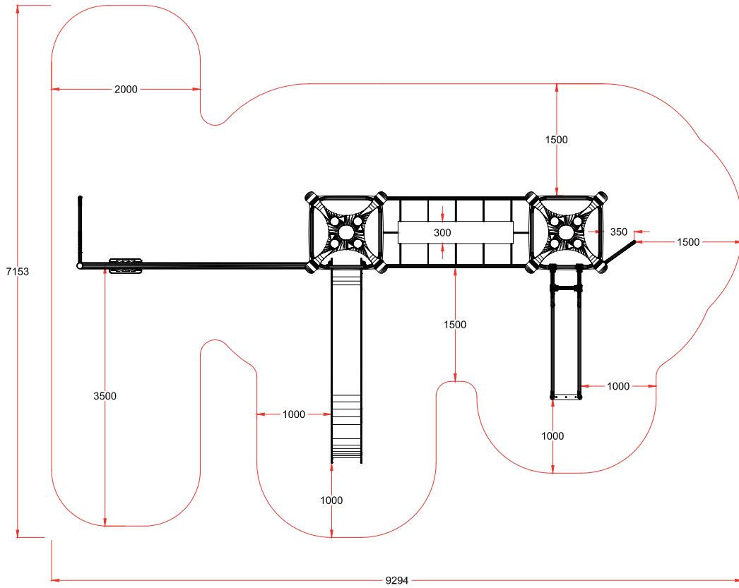
PLANTA CIMENTACION
