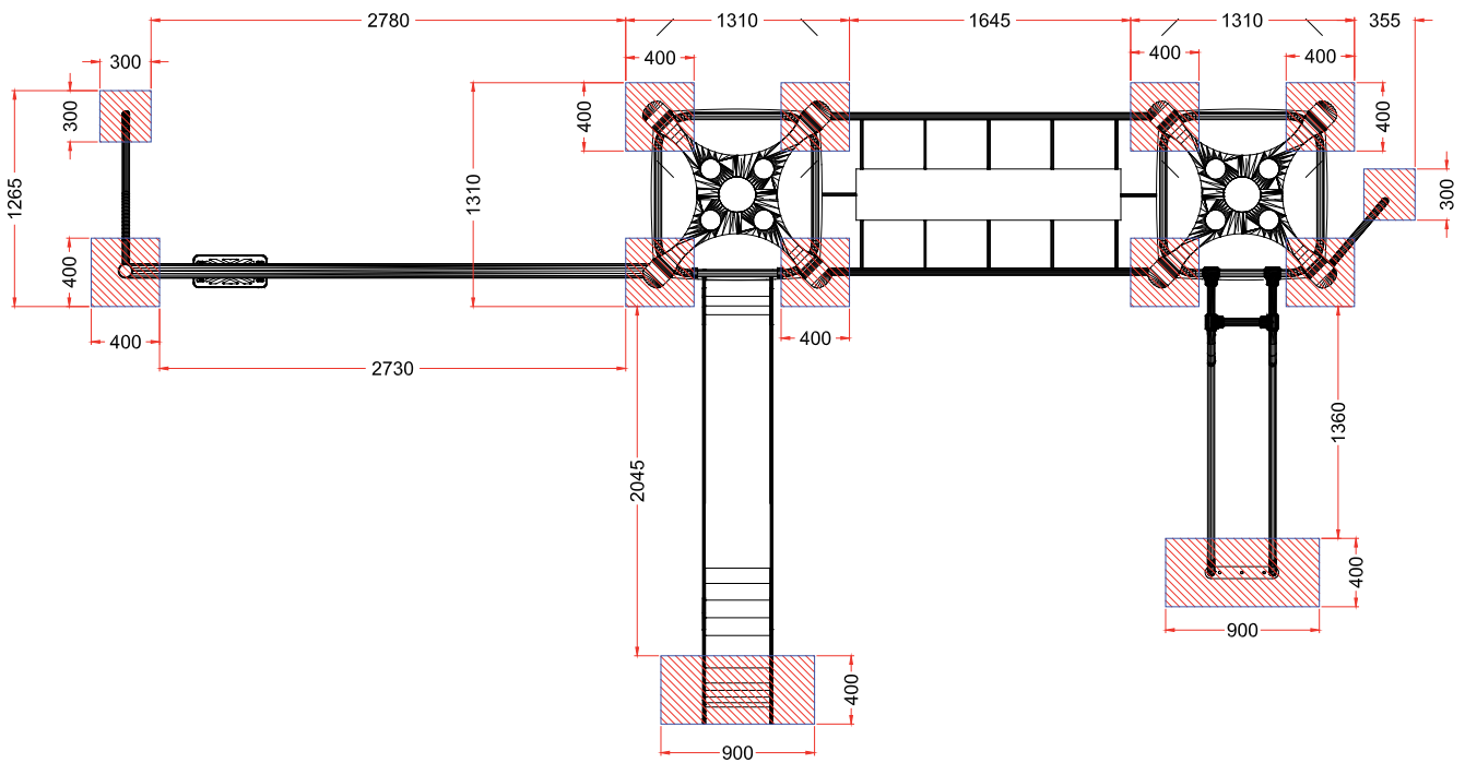
PLANTA CIMENTACION
