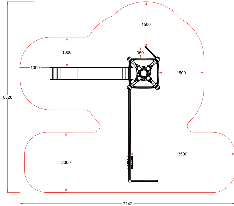
PLANTA
