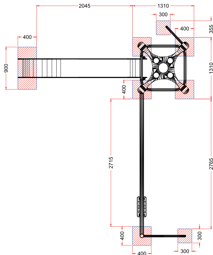
PLANTA CIMENTACION
